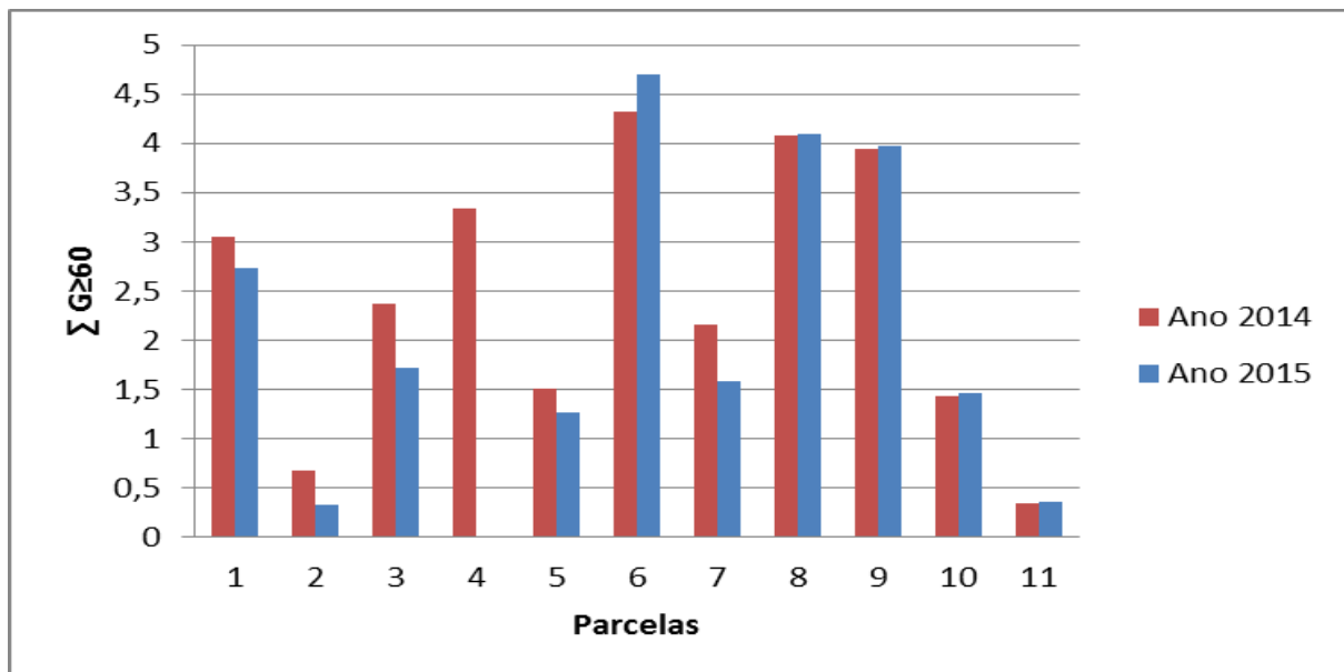
Figura 4. Distribuição da área basal remanescente ao longo das parcelas no experimento da EMBRAPA, Km 67 da Flona do Tapajós para \Sigma G \geq 60 ( m^2/ha ). Valores calculados para indivíduos com DAP > 60 cm em 2014 e 2015.
