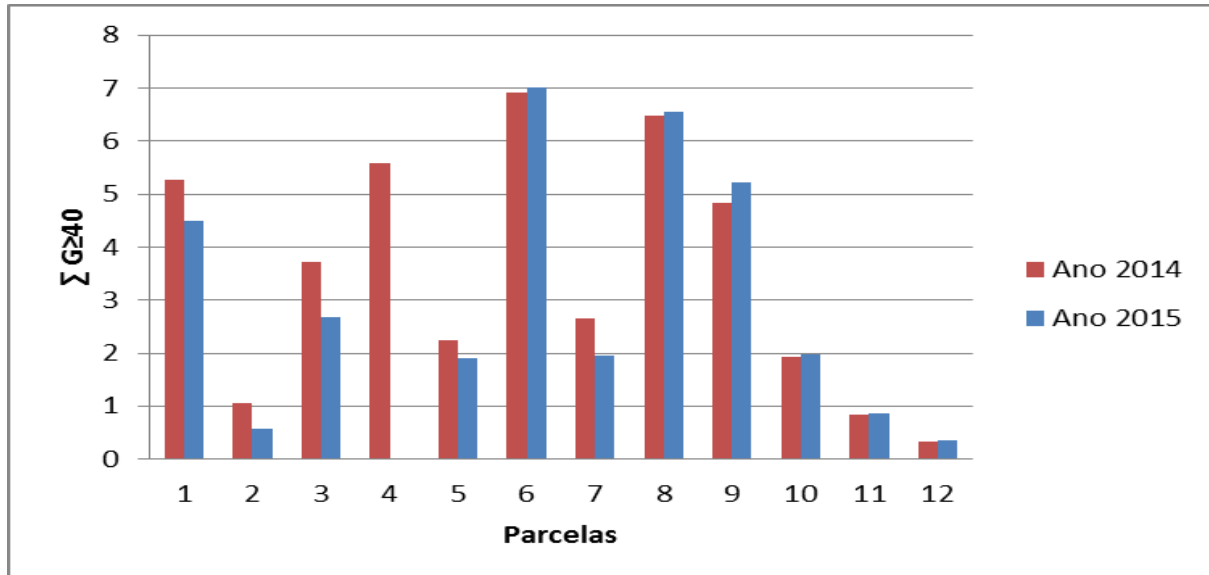
Figura 3. Distribuição da área basal remanescente ao longo das parcelas no experimento da EMBRAPA, Km 67 da Flona do Tapajós para \Sigma G \geq 40 ( m^2/ha ). Valores calculados para indivíduos com DAP > 40 cm em 2014 e 2015.
