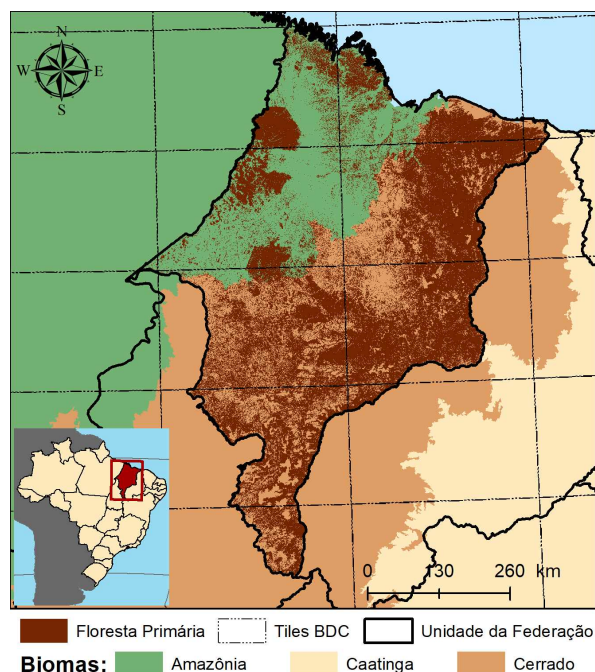
Figura 1: Localização da área de estudo, com destaque para os tiles do BDC.
