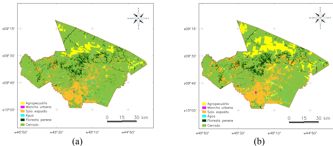
Figura 2: Mapa de cobertura da terra da área de estudo em 1999 (a) e 2009 (b).
