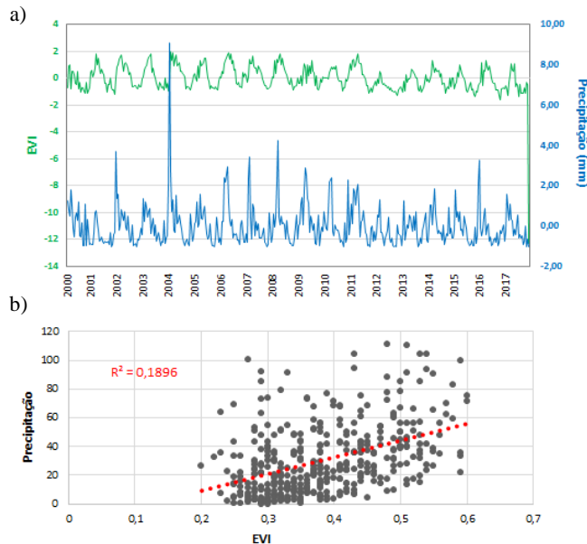
Figura 2. Gráfico de resposta multitemporal (a) e gráfico de dispersão (b) do EVI e Precipitação no bioma Caatinga em áreas de vegetação natural.
