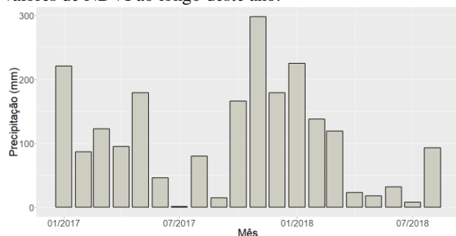
Figura 3. Precipitação média mensal na área de estudo.
