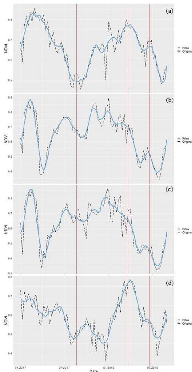
Figura 2. Série temporal do NDVI para os talhões: (a) fazenda 1 - talhão 2; (b) fazenda 1 - talhão 10, piquete 1; (c) fazenda 1 - talhão 10, piquete 2; e (d) fazenda 2 - talhão 1. As linhas verticais em vermelho correspondem às datas das visitas a campo.
