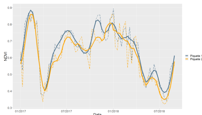
Figura 4. Série temporal do NDVI para dois piquetes do talhão 10 da fazenda 1. As linhas tracejadas representam a série original e as linhas cheias com o filtro.
