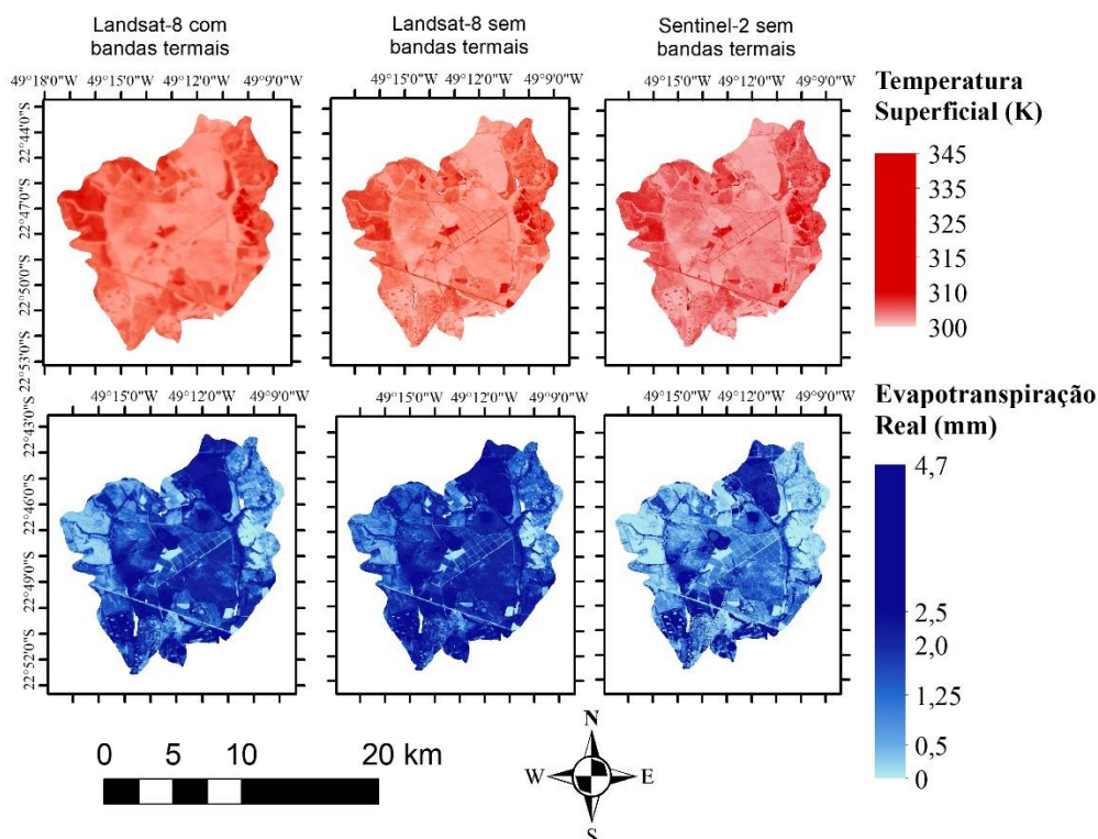
Figura 2. Distribuição espacial da temperatura superficial e evapotranspiração real no dia 26 de novembro de 2016 obtidos com imagens dos satélites Sentinel-2 e Landsat-8 e dados agrometeorológicos.
