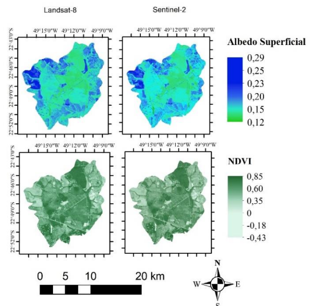
Figura 1. Distribuição espacial do albedo superficial e NDVI no dia 26 de novembro de 2016 obtidos com imagens dos satélites Sentinel-2 e Landsat-8.
