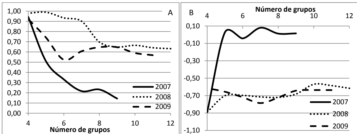
Figura 4. (A) Gráfico do coeficiente de correlação linear entre índice de dengue e a densidade populacional versus o número de grupos gerados. (B) Gráfico do coeficiente de correlação linear entre índice de dengue e o percentual de domicílios sem ligação de água versus o número de grupos gerados.
