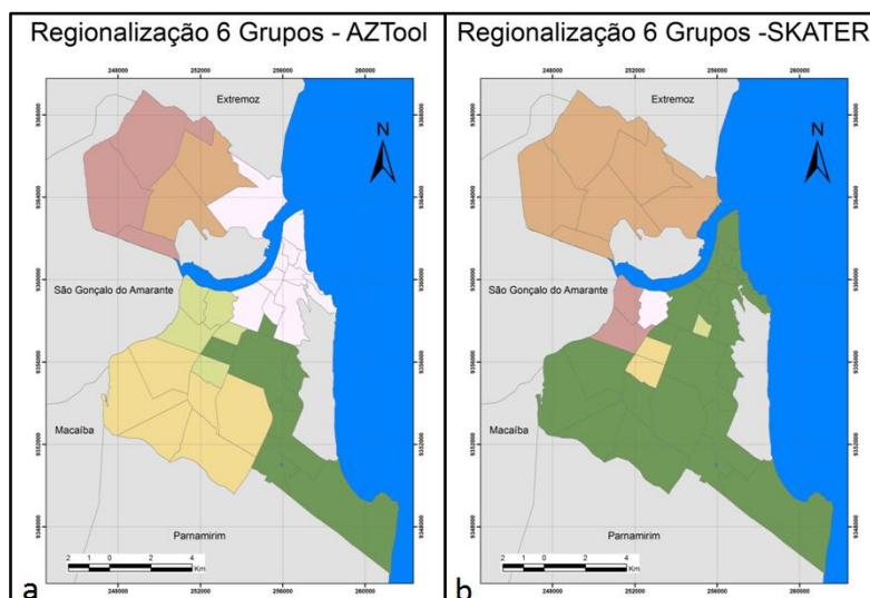
Figura 5. Dois cenários diferentes para a escala de agregação em seis grupos obtida com a metodologia AZTool (a) e a SKATER (b).
