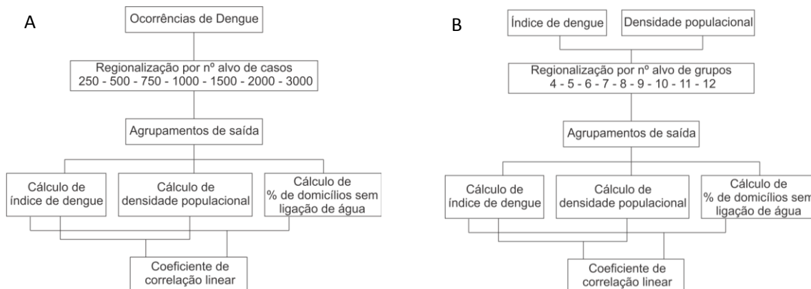
Figura 2. (A) Fluxograma da metodologia de regionalização AZTool. (B) Fluxograma da metodologia de regionalização SKATER.
