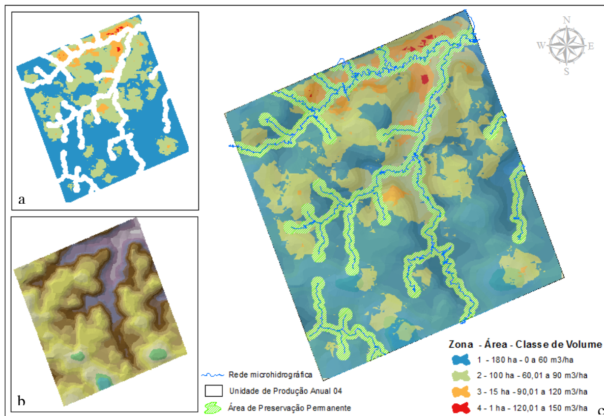
Figura 5. a) Imagem raster de volumetria reclassificada e sem influência da APP; b) Modelo Digital do Terreno gerado a partir da imagem SRTM e; c) Proposta de Unidades de Gestão Diferenciada (Zonas).
