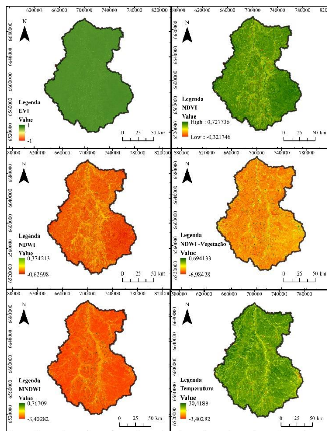
Figura 8 - Resultados para evi, ndvi, ndwi, mndwi, ndwi-veg e temperatura na bacia hidrográfica do rio santa maria.
